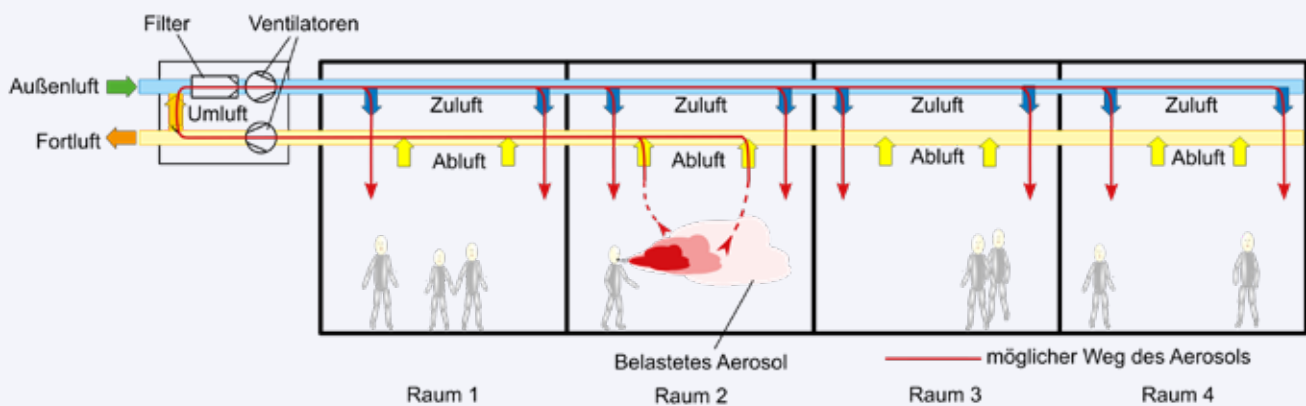
Abbildung 1: Zentrale Klimaanlage
